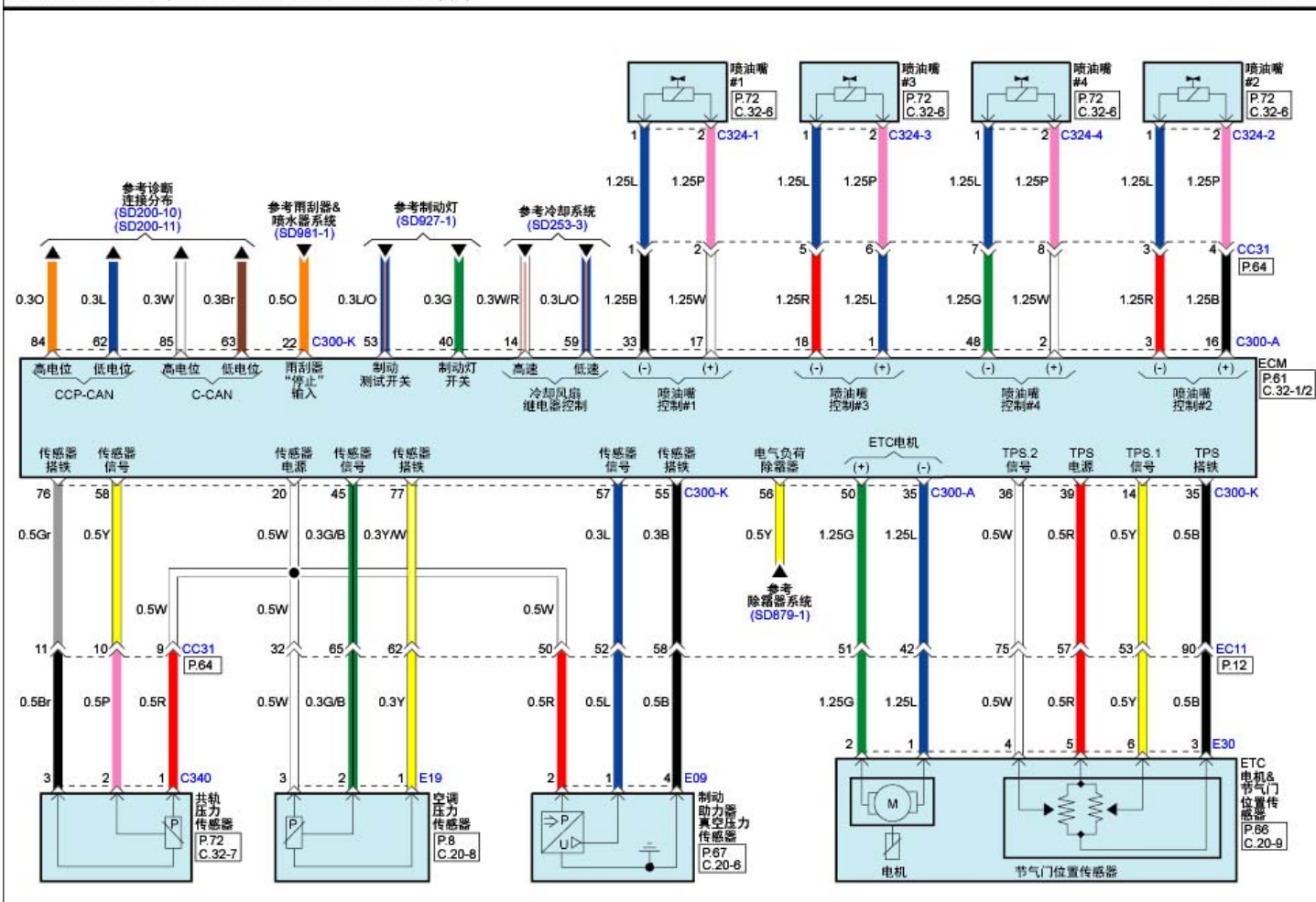
发动机控制系统(G4FJ : GAMMA 1.6L T-GDI)(7)
